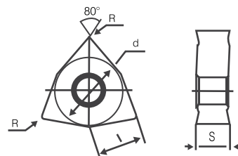
Forma WNMG
